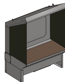
UF-EM Bagvæg med skrå top med sug 30° vinklet, lys i top, lameller langs sider samt on/off-kontakt for lys i bord. Standard med stålribber.
