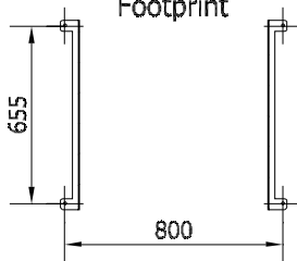
A-A ( 1 : 25 ) Footprint
